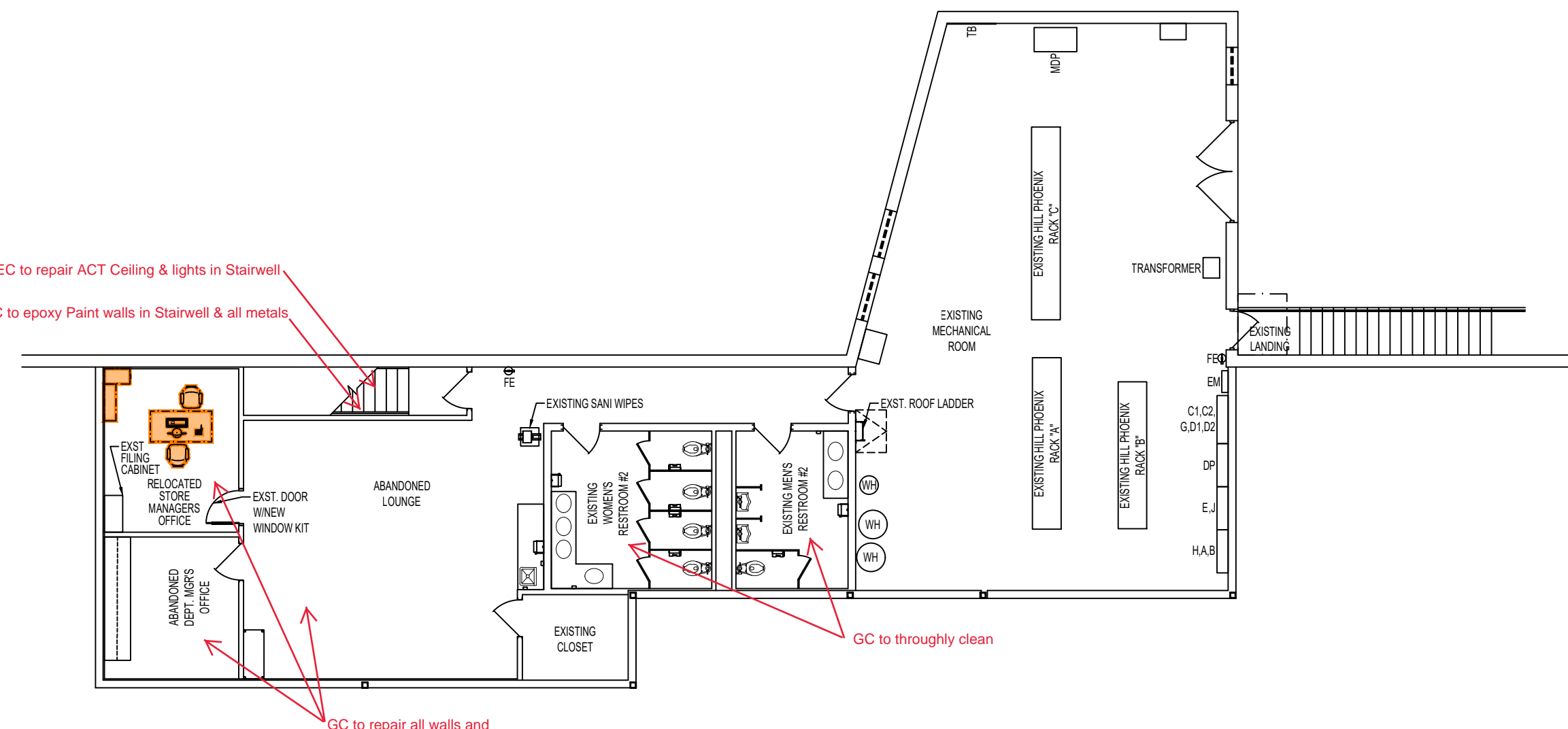
MEZZANINE SCALE: 3/32" = 1'-0"
